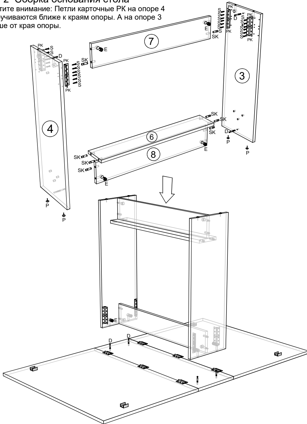
Рис. 2 Сборка основания стола
